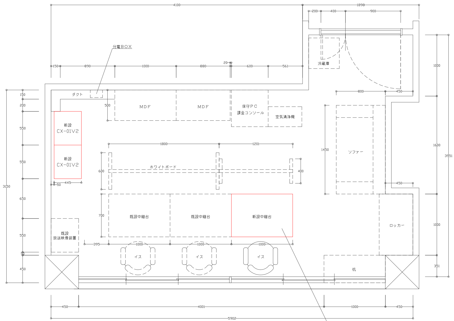
施工完了後(案)一平面図
