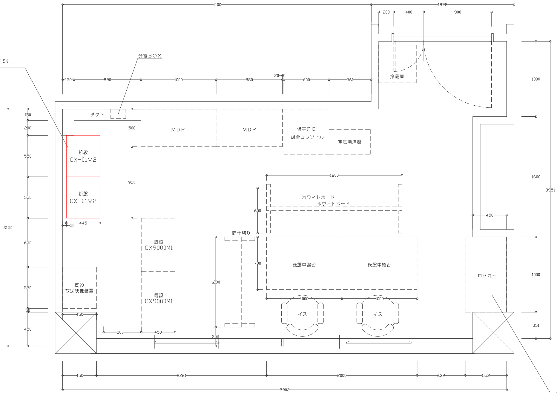
仮設置(案)一平面図
