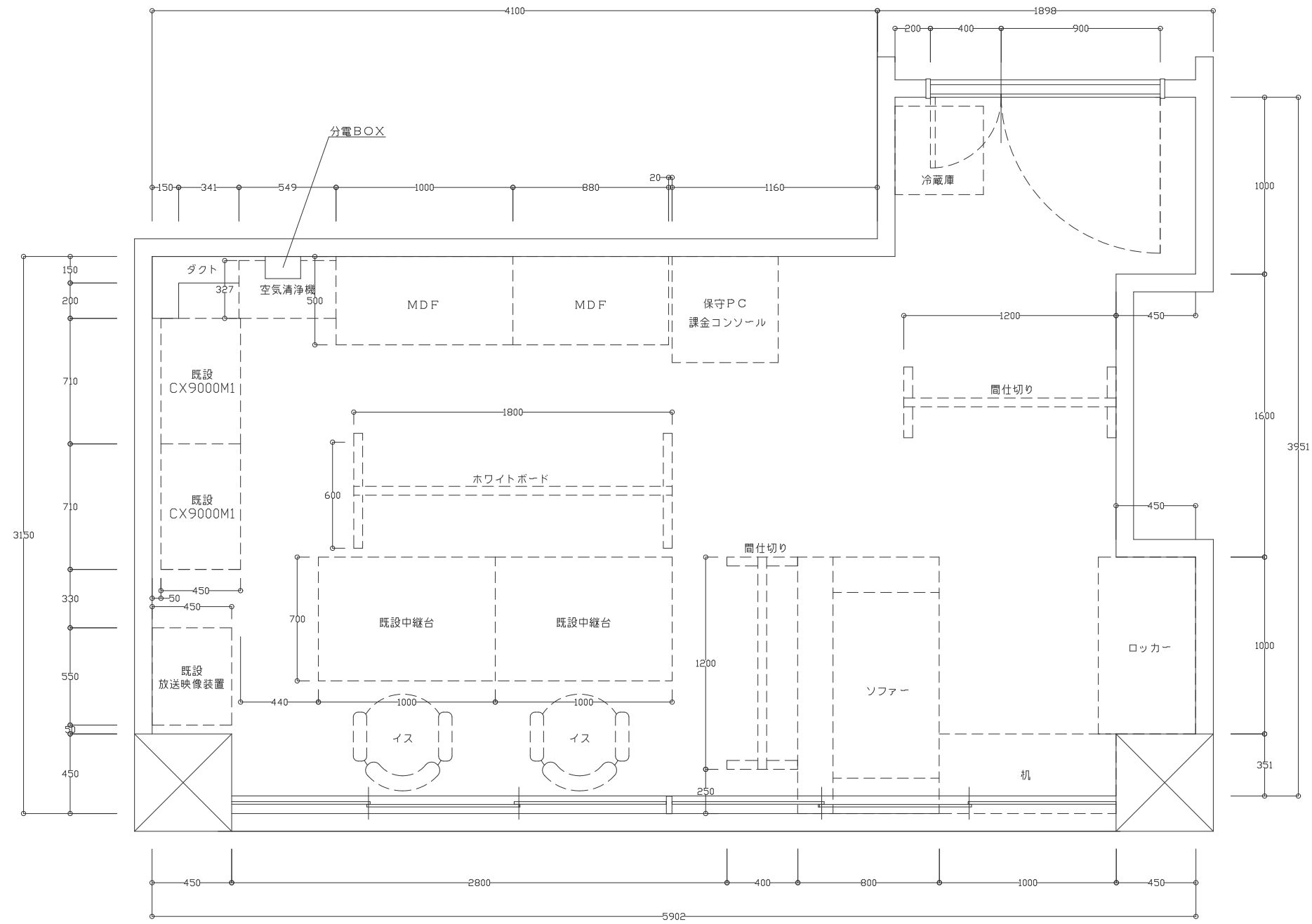
現状図一平面図
